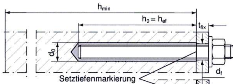
Ankerstange Vorsteckmontage
