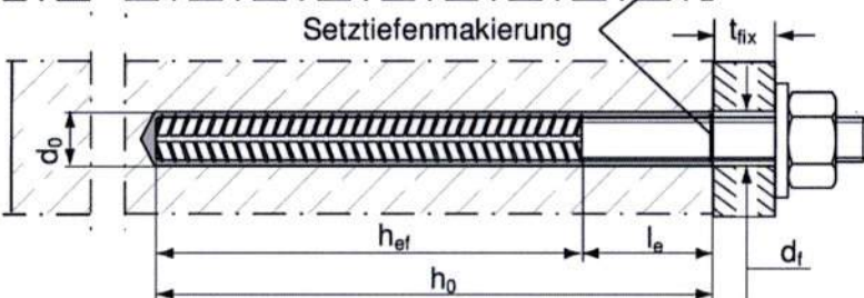
fischer Bewehrungsanker FRA Vorsteckmontage
